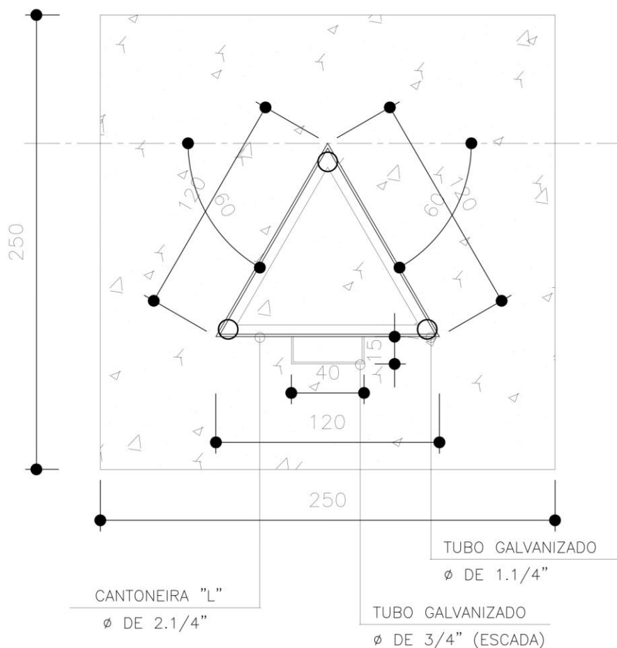
DETALHE DA BASE ESCALA 1/20
